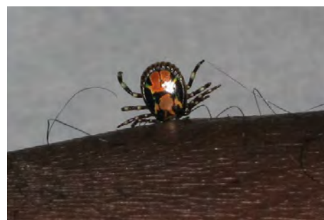
Tique, vectrice de la bactérie Borrelia , responsable de la maladie de Lyme
